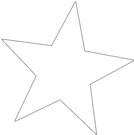
star
