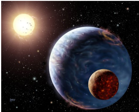
planet
